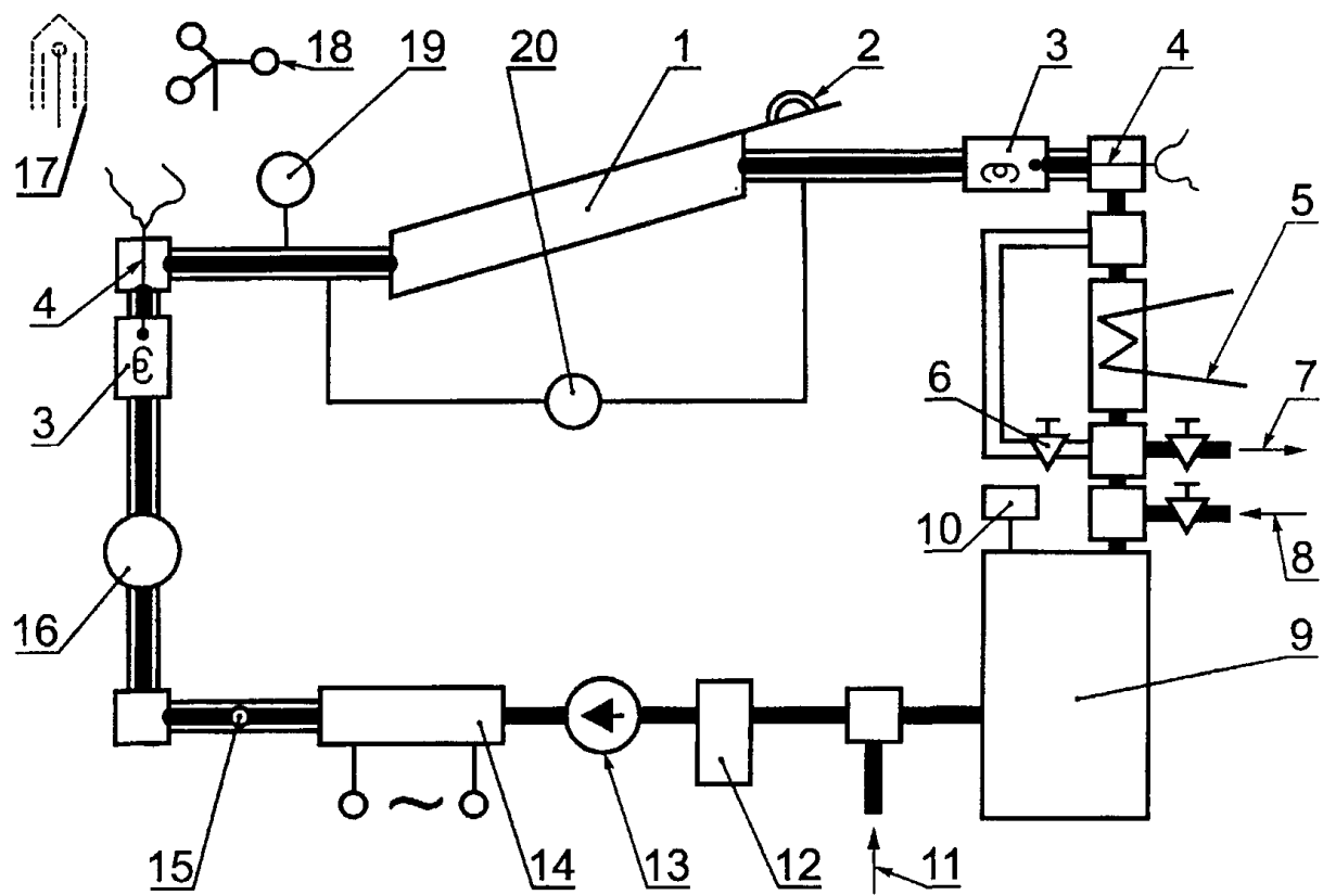
1 — испытуемый СК; 2 — пиранометр; 3 — камера смешения; 4 — датчик температуры теплоносителя; 5 — теплообменник; 6 — байпасный вентиль; 7 — вывод теплоносителя на очистку; 8 — ввод теплоносителя после очистки; 9 — накопительный бак; 10 — расширительный бак с предохранительным клапаном; 11 — ввод теплоносителя в контур; 12 — фильтр; 13 — циркуляционный насос; 14 — регулируемый электронагреватель; 15 — смотровое стекло; 16 — расходомер; 17 — датчик температуры окружающего воздуха; 18 — анемометр; 19 — манометр; 20 — дифманометр
