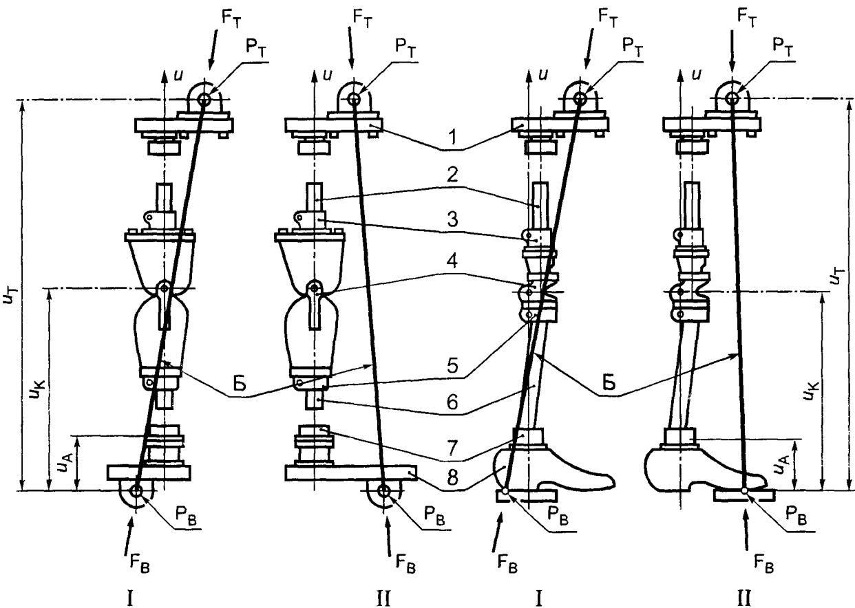
I, II — условия нагружения; Б — линия нагружения; 1 — верхний нагрузочный рычаг; 2 — удлинитель; 3 — соединитель (переходник); 4 — коленный узел; 5 — соединитель (переходник); 6 — удлинитель; 7 — переходник (голеностопный узел); 8 — нижний нагрузочный рычаг (стопа)
