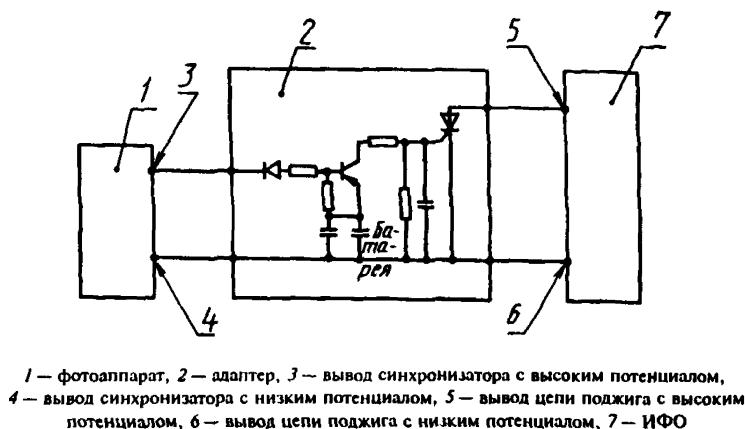
Рисунок В.5 — Примерная схема адаптера
