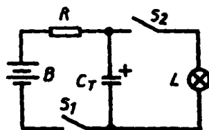
Рисунок В.3 — Пример цепи поджига типа В
