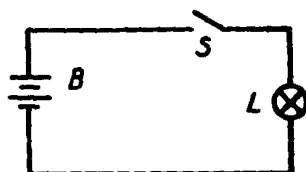
Рисунок В.3 — Пример цепи поджига типа В
