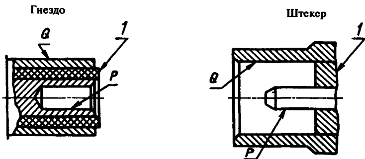
Рисунок 2 — Полярность гнезда и штекера в миниатюрных штепсельных соединителях портативных фотоаппаратов
