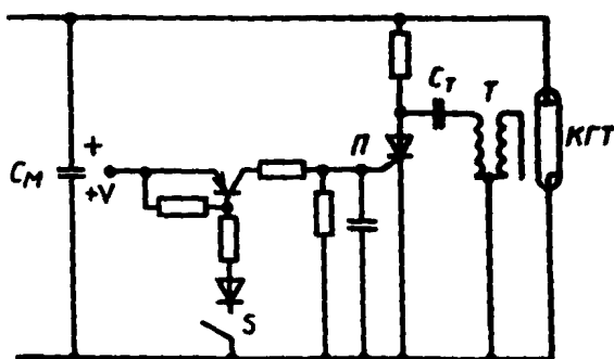
Рисунок В.2 — Пример цепи поджига полупроводникового типа
