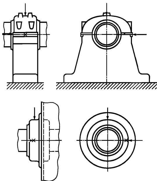
Рисунок 1 — Точки измерений на коренных подшипниках
