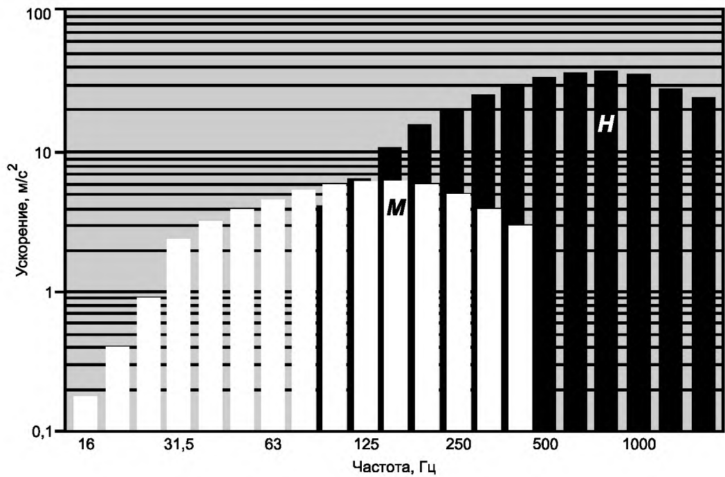
Рисунок С.1 — Спектры М и Н
