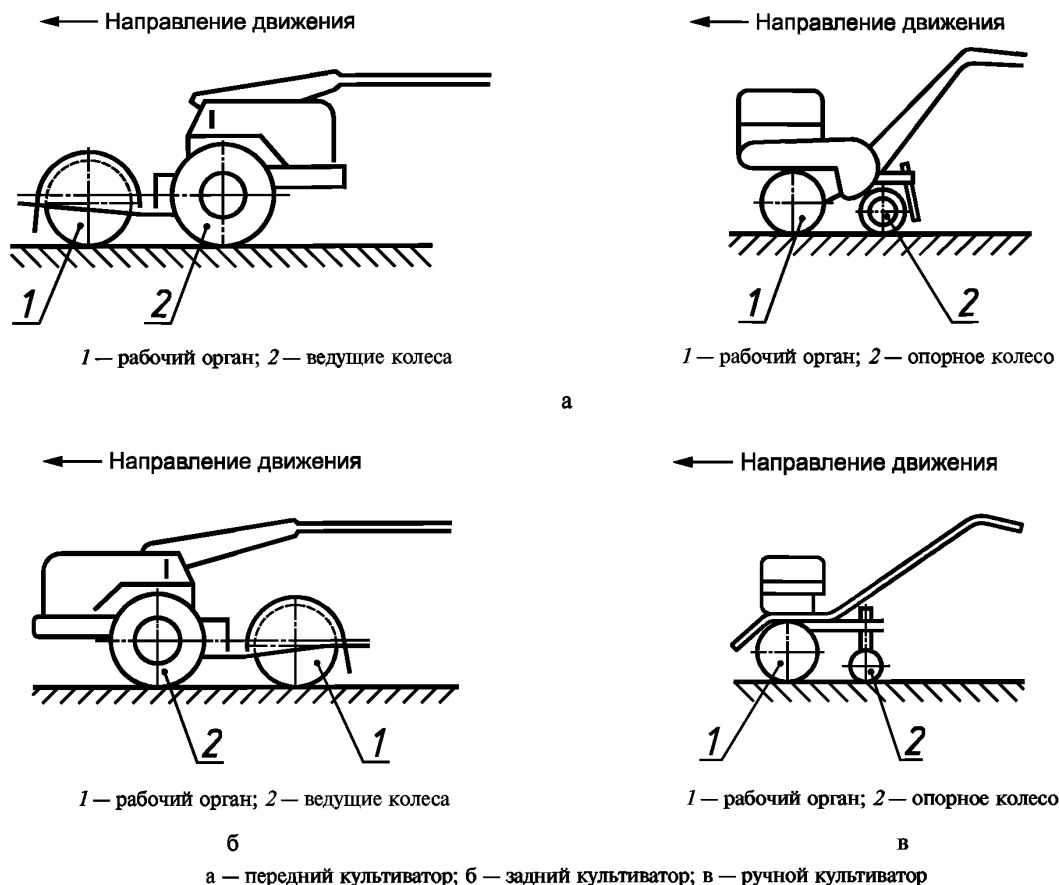
Рисунок 1 — Типы культиваторов
