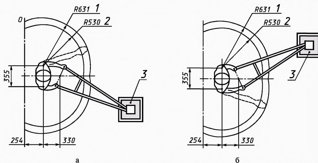
Рисунок 5 — Зона оператора, идущего рядом с культиватором
