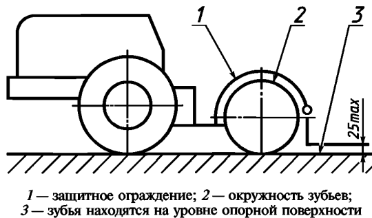
Рисунок 2 — Защита рабочего органа заднего культиватора
