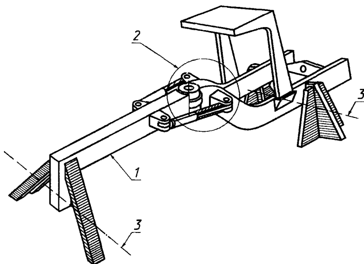
Рисунок 8 — Закрепление автогрейдера с шарнирно-сочлененной рамой
