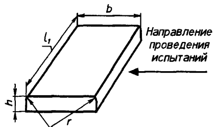
Рисунок 1 — Препятствие для проведения испытаний
