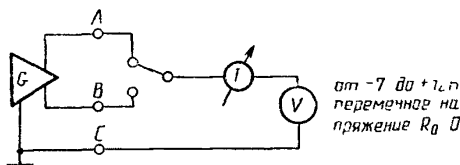
Рисунок 14 Проверка соперничества генераторов
