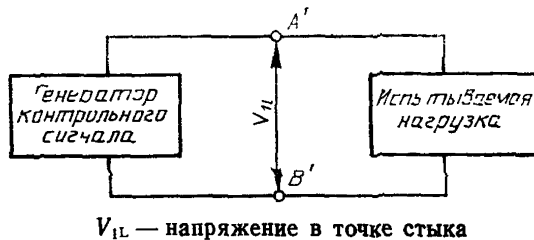
Рисунок 6 — Испытательная схема нагрузки V.11
