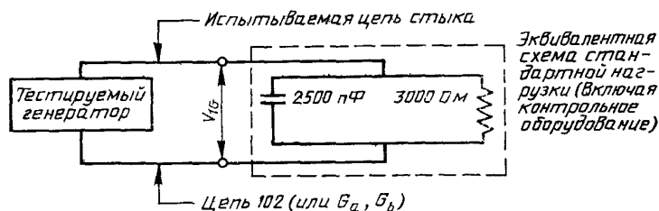
Рисунок 1 — Испытательная схема генератора V.28
