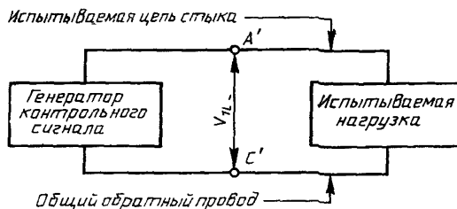
Рисунок 4 — Испытательная схема нагрузки V.10
