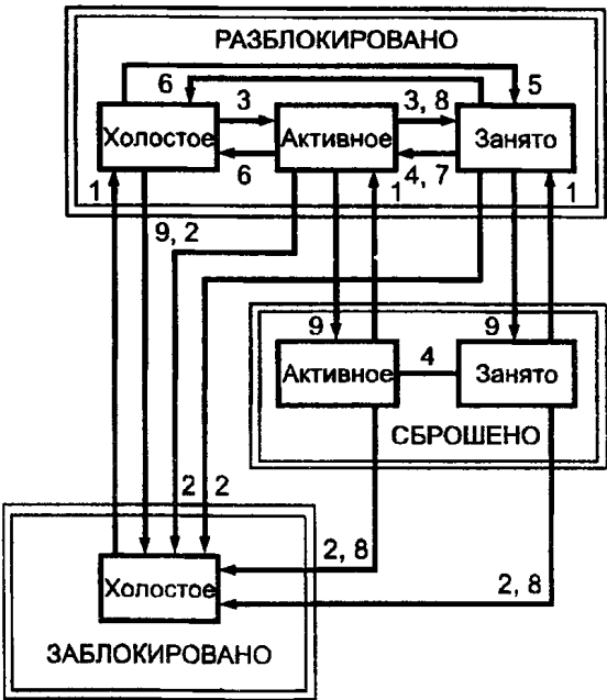
Рисунок 5 — Рабочее и административное состояния
