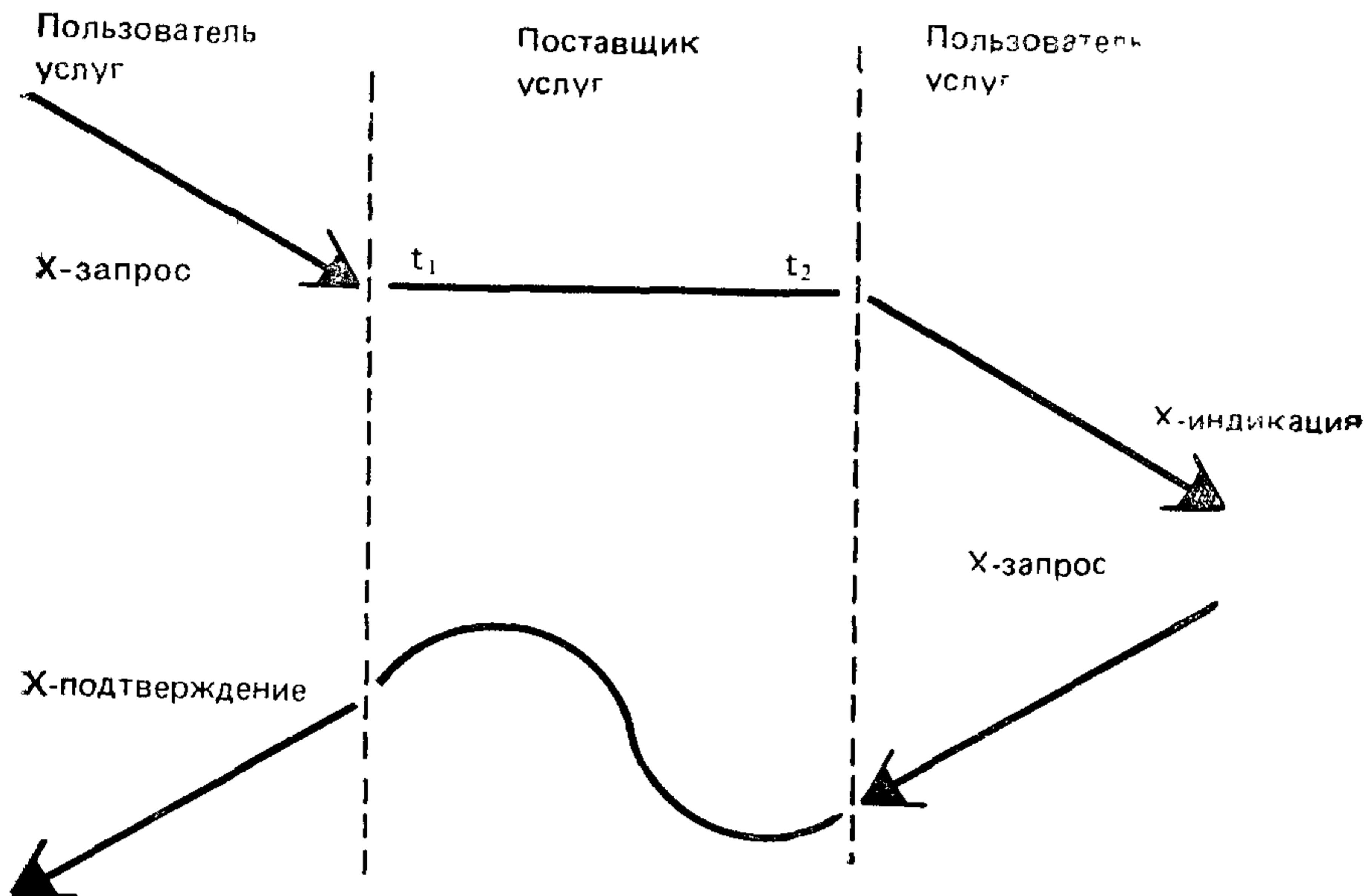
Рисунок 3 — Пояснения к временным диаграммам
