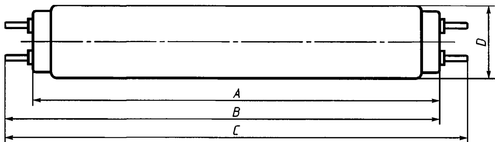
Цоколи G5 и G13 по МЭК 60061-1
