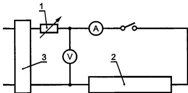
Рисунок А.5 — Схема испытания на зажигание ламп без предварительного подогрева катодов для работы на ВЧ
