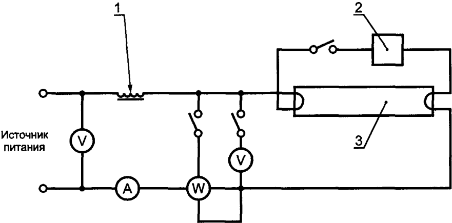
1 — образцовый ПРА; 2 — стартер; 3 — лампа
