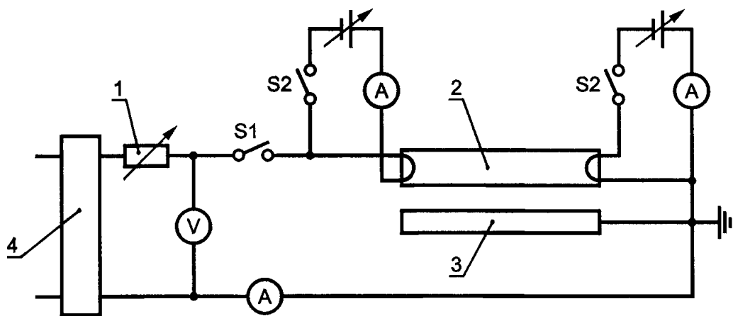
1 — резистор; 2 — лампа; 3 — ЗВУ; 4 — ВЧ генератор
