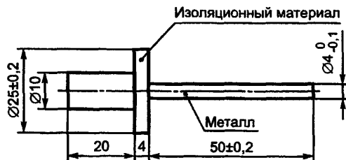
Рисунок 104 — Длинный испытательный шуп
