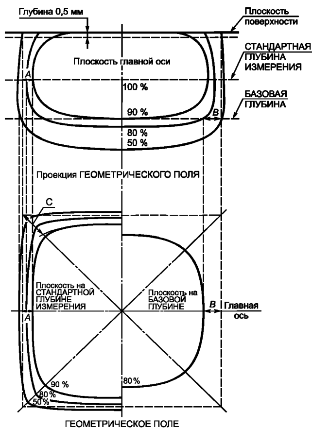
Рисунок 6 — Примеры диаграммы равномерности ЭЛЕКТРОННОГО ПОЛЯ
