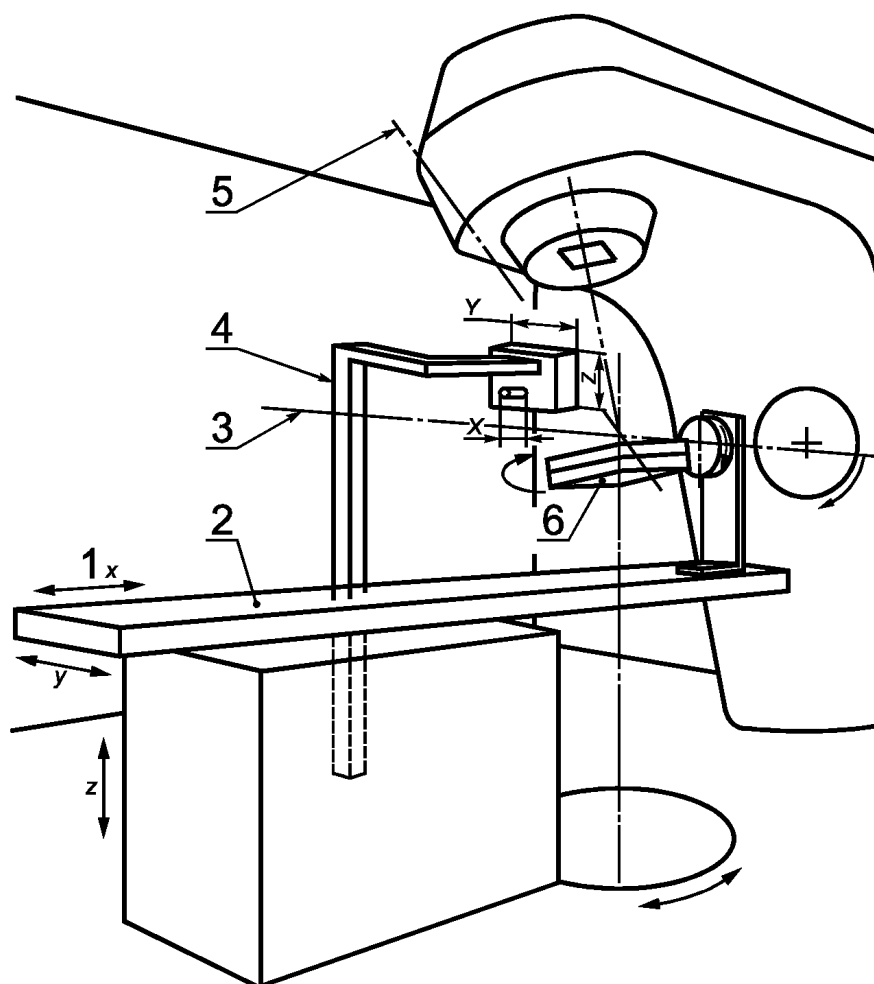
1 — x, y, z — микрометрическая настройка опорного указателя; 2 — дека СТОЛА для ПАЦИЕНТА; 3 — настенный источник света; 4 — держатель центратора, укрепленный на полу, позволяющий поворачивать ШТАТИВ на 360^\circ и СТОЛ для ПАЦИЕНТА на меньшие углы; 5 — потолочный источник света; 6 — блок из моделирующего материала и пленка
