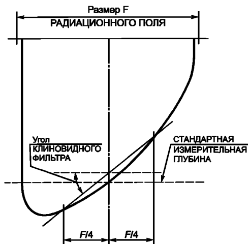
Рисунок 7 — Пояснение к определению УГЛА КЛИНОВИДНОГО ФИЛЬТРА
