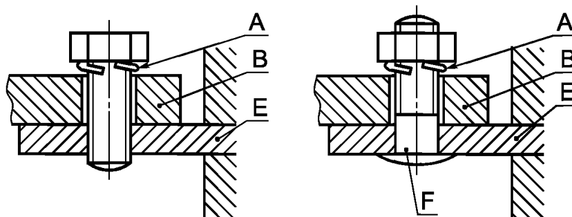
Рисунок 4 — Примеры зажимов под наконечник
