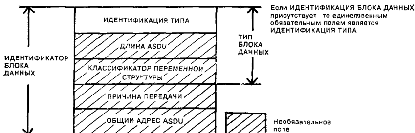
Рисунок 7 — Основная структура ИДЕНТИФИКАТОРА БЛОКА ДАННЫХ
