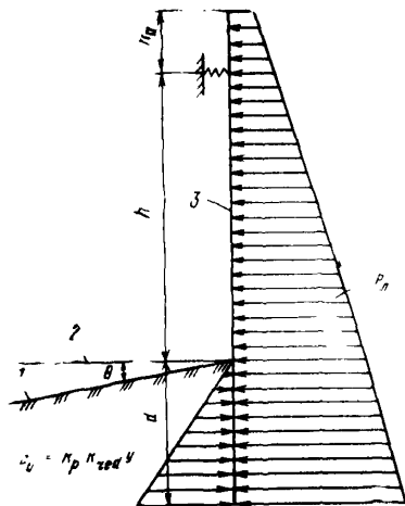
Рис. 5.1. Расчетная схема лицевой стенки существующего бойлера: 1 — проектное дно; 2 — существующее дно; 3 — расчетная плоскость
