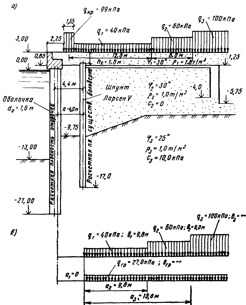
Рис. 3. Схема сооружения: а — конструктивная схема; б — схема расположения вертикальных нагрузок за расчетной плоскостью существующего бойлерка
