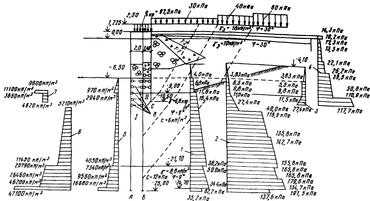
Рис. 2. Расчетная схема:
