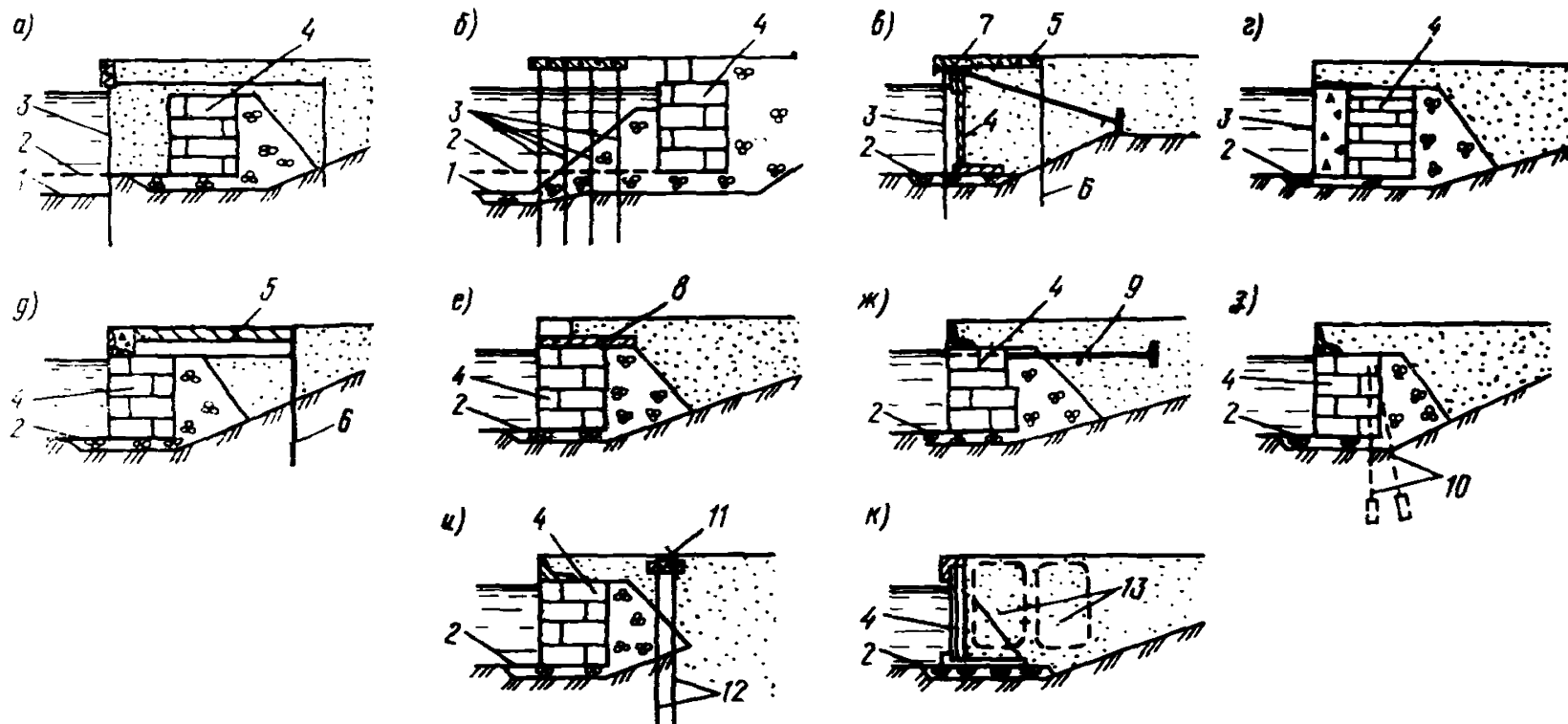
Рис. 3.4. Схемы реконструкции и усиления гравитационных сооружений путем устройства:
