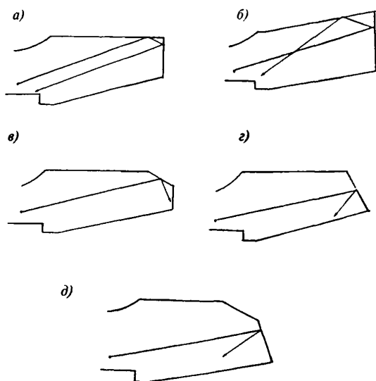
а и б — «театральное эхо», в — г — «театральное эхо» отсутствует
