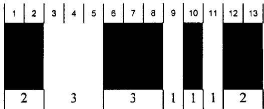
Рисунок 4 — Знак Stop для Code 128
