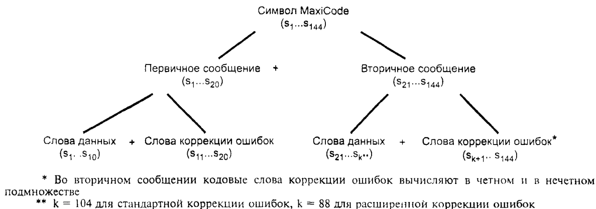
Рисунок 6 — Структура символа и обозначения знаков символа
