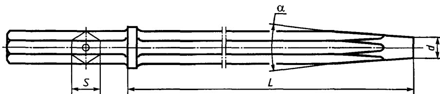
Рисунок 1 — Буровые штанги с конусом
