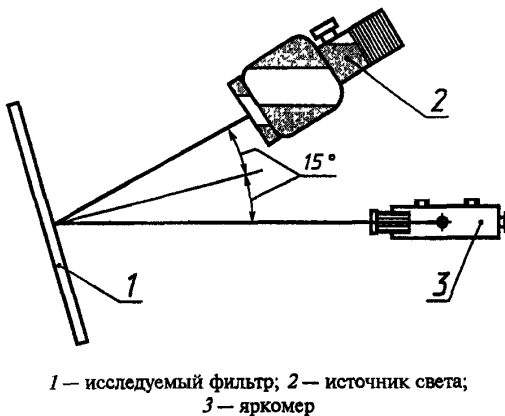
Рисунок 3 — Схема измерения коэффициента зеркального отражения фильтра в видимом диапазоне длин волн
