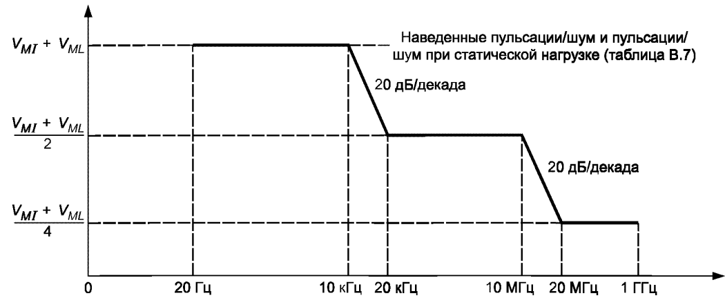
Рисунок В.44 — Пределы пульсаций/шума наведенной помехи и помехи при статической нагрузке базового блока
