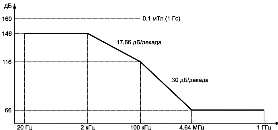
Рисунок В.48 — Максимальные уровни помех ближнего поля для модулей типов С и D (дБ относительно 1 пТл)
