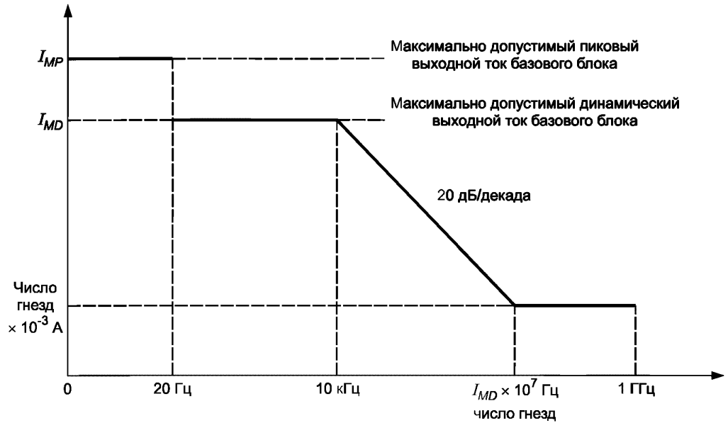
Рисунок В.43 — Ток нагрузки базового блока
