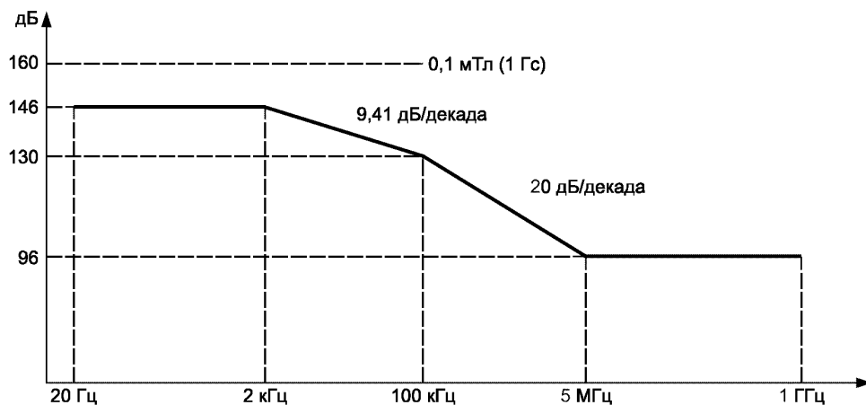
Рисунок В.47 — Максимальные уровни помех ближнего поля для модулей типов А и В (дБ относительно 1 пТл)
