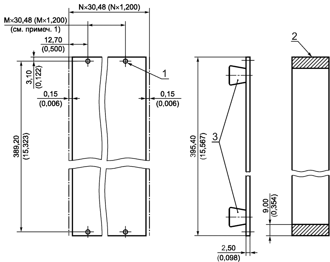
1 — см. рисунок В.23; 2 — минимальная зона корпусного электроконтакта; 3 — см. примечание 2
