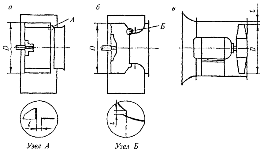
Рис. 2. Схемы зазоров вентиляторов: a — радиальных типа В.Ц14-46; б — радиальных типа В.Ц4-70; в — осевых ( z=0,5-1,0\%D )
