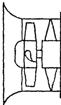
Рис. 1. Схемы конструктивных исполнений вентиляторов: а — радиальных; б — осевых
