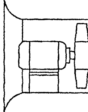
Рис. 1. Схемы конструктивных исполнений вентиляторов: а — радиальных; б — осевых
