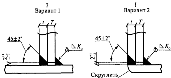
Рис. 3.10. Люк-лаз круглый в I поясе стенки
