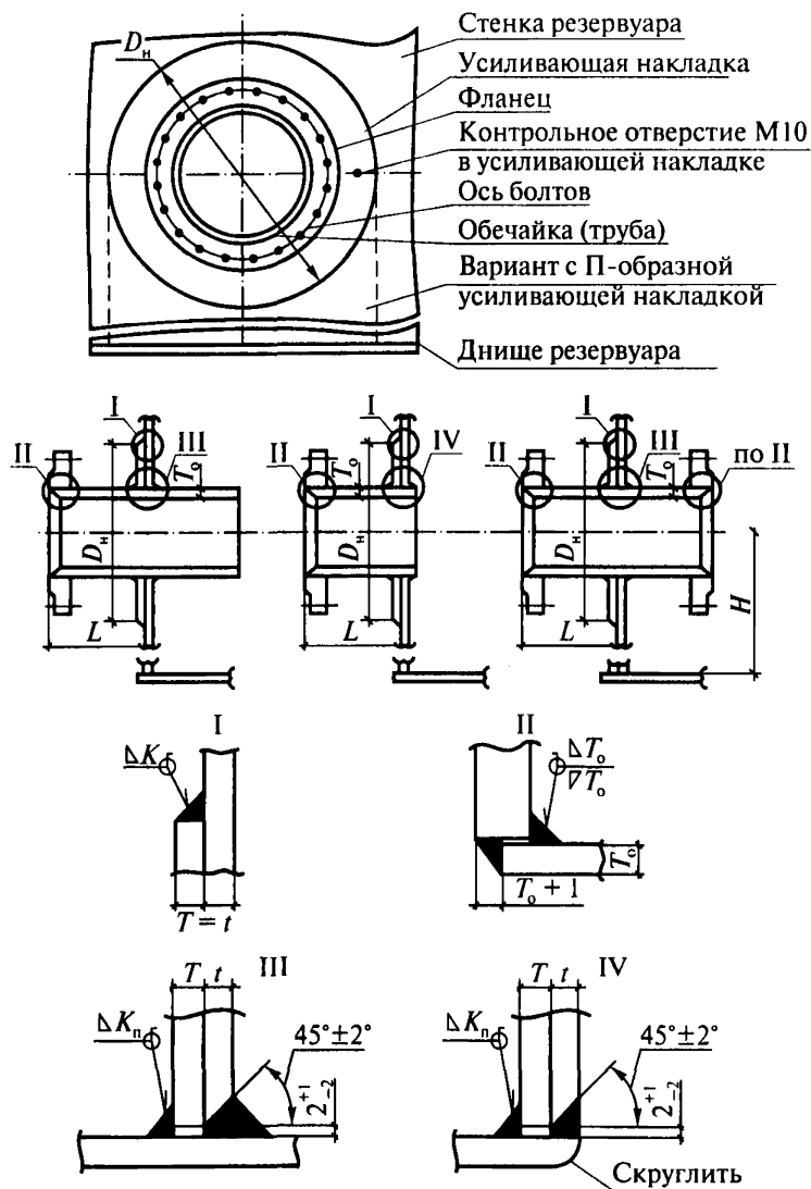
Рис. 3.9. Общий вид патрубка в стенке резервуара
