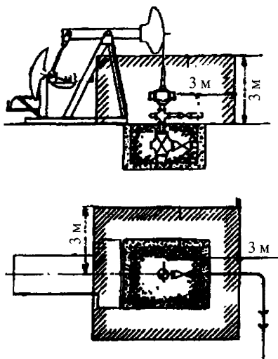
Рис. 5. Открытые пространства вокруг фонтанных арматур
