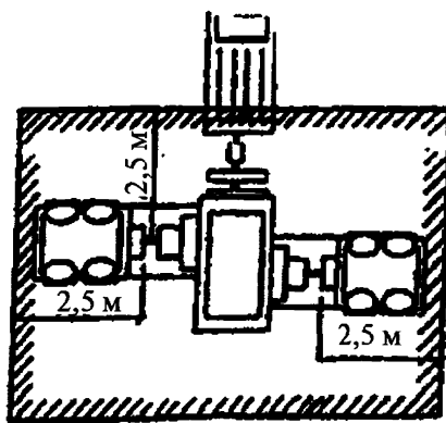
Газовый компрессор
