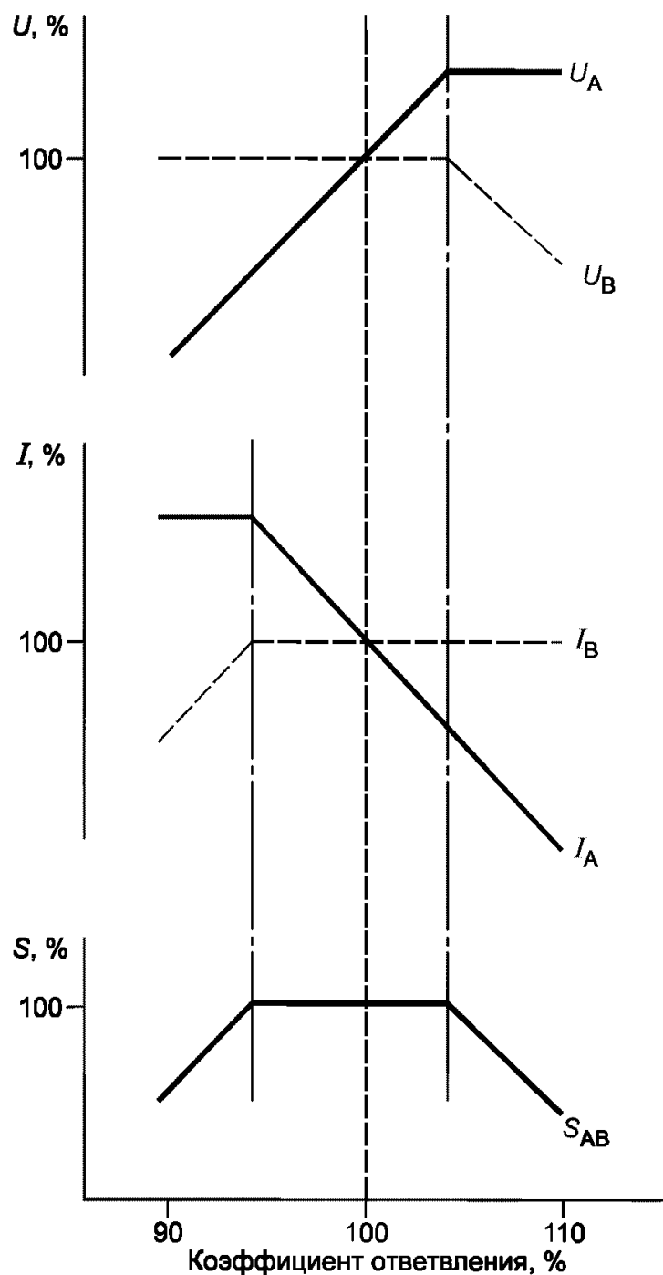
Рисунок 3 — Комбинированное регулирование напряжения (режим е )
