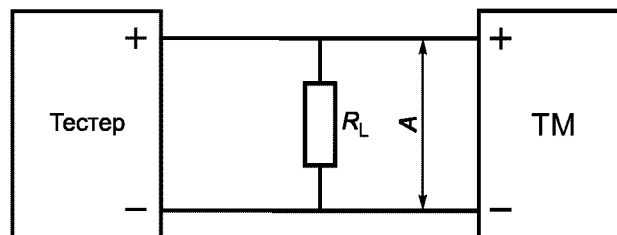
Рисунок 1 — Общая схема тестирования
