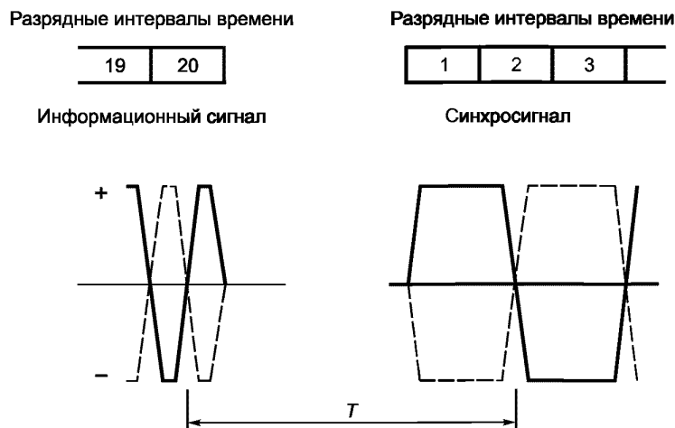
Рисунок 6 — Измерение временных пауз при передаче информации
