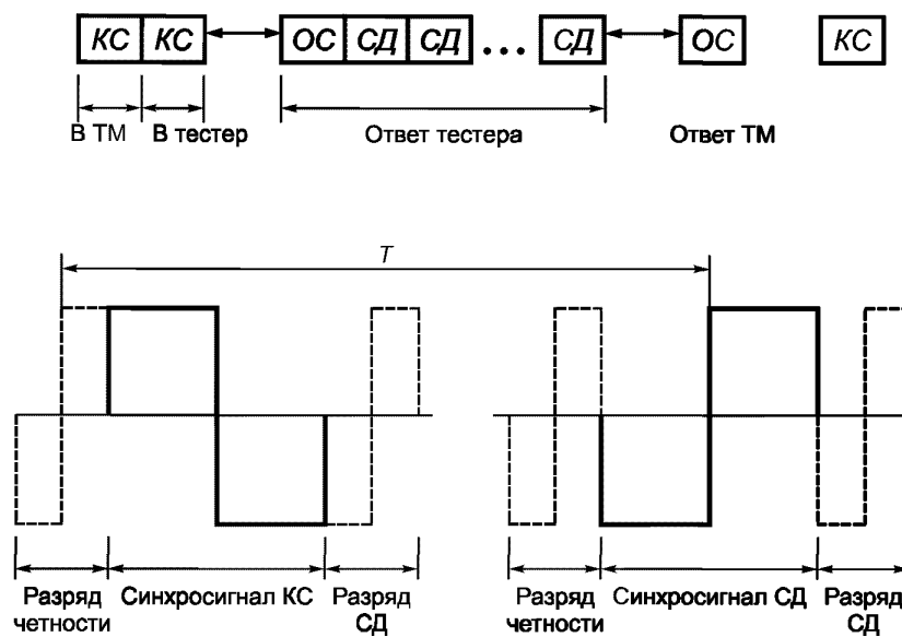
Рисунок 7 — Измерение времени тайм-аута при передаче сообщений в формате ОУ-ОУ
