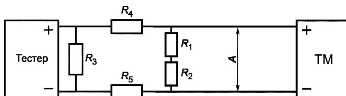
Рисунок 2 — Схема тестирования
