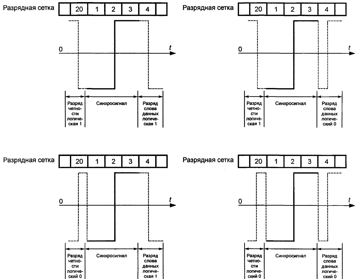
Рисунок 7 — Синхросигналы слов данных
