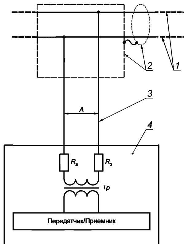
Tr — трансформатор гальванической развязки; R_3 — защитные резисторы; 1 — магистральная шина; 2 — экран; 3 — шлейф; 4 — устройство интерфейса
