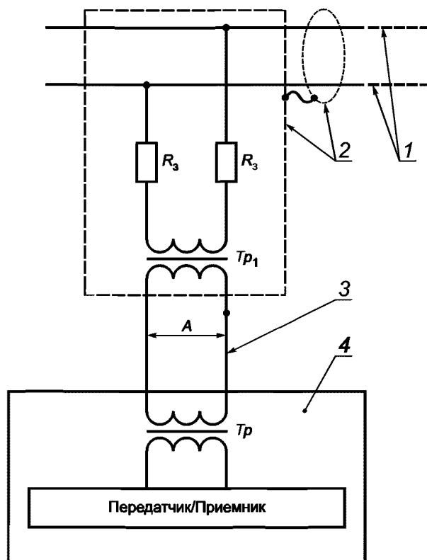
Tr — трансформатор гальванической развязки; Tr_1 — согласующий трансформатор; R_3 — защитные резисторы; 1 — магистральная шина; 2 — экран; 3 — шлейф; 4 — устройство интерфейса
