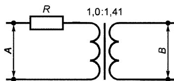
Рисунок 11 — Согласующий трансформатор
