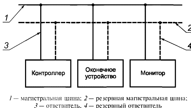
Рисунок 1 — Структурная схема технических средств интерфейса
