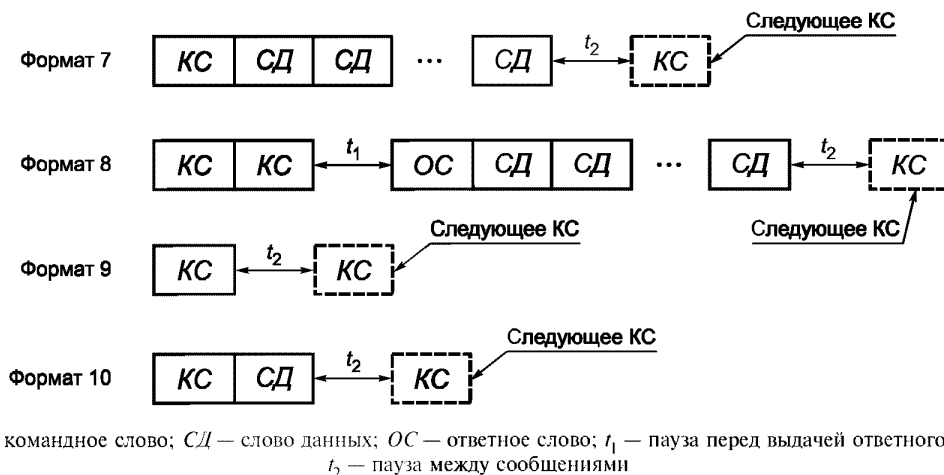
Рисунок 9 — Форматы групповых сообщений
