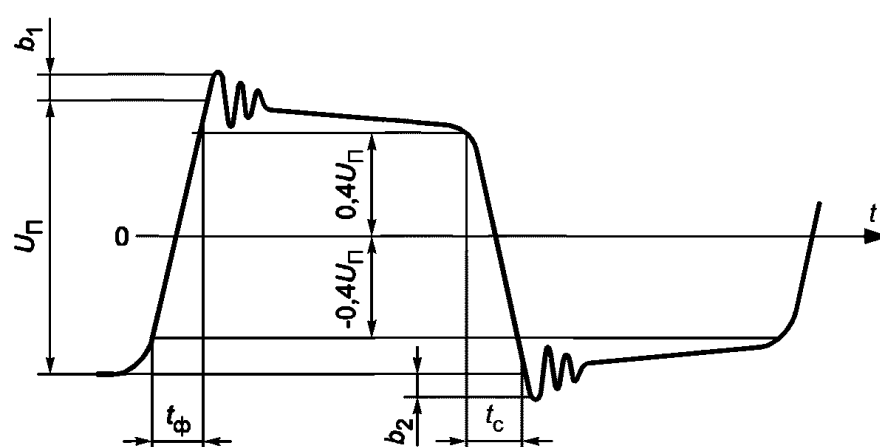
Рисунок 15 — Форма выходного сигнала устройства интерфейса
