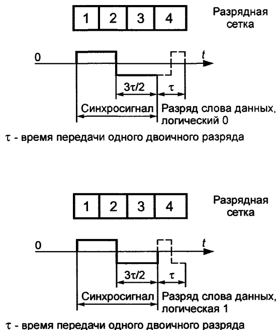
Рисунок 4 — Синхросигнал командного и ответного слов
