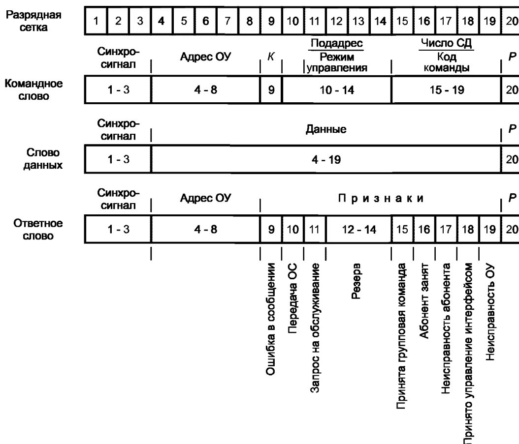
Рисунок 3 — Форматы передаваемых слов
