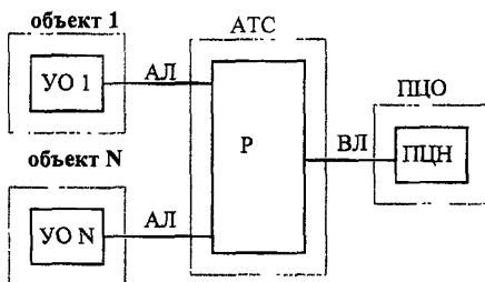
Рисунок 5.1 - Структура СПИ
