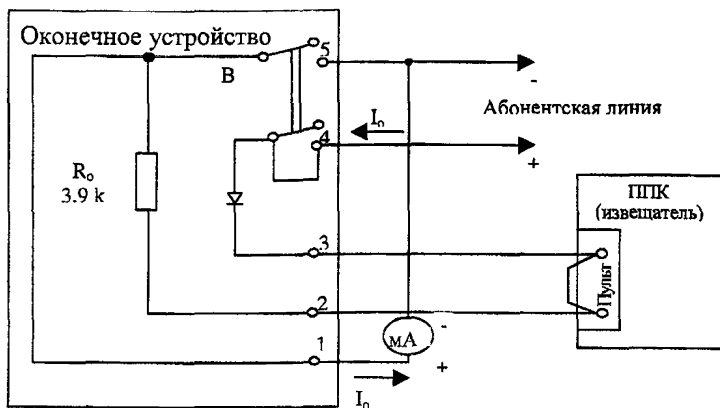
Рисунок П 1.3 - Схема измерения тока систем "Нева-10М" и "Нева"
