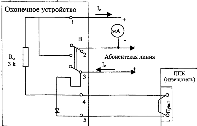
Рисунок П 1.1. – Схема измерения тока системы "Центр-М"
