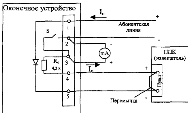
Рисунок П 1.2- Схема измерения тока системы "Центр-КМ"
