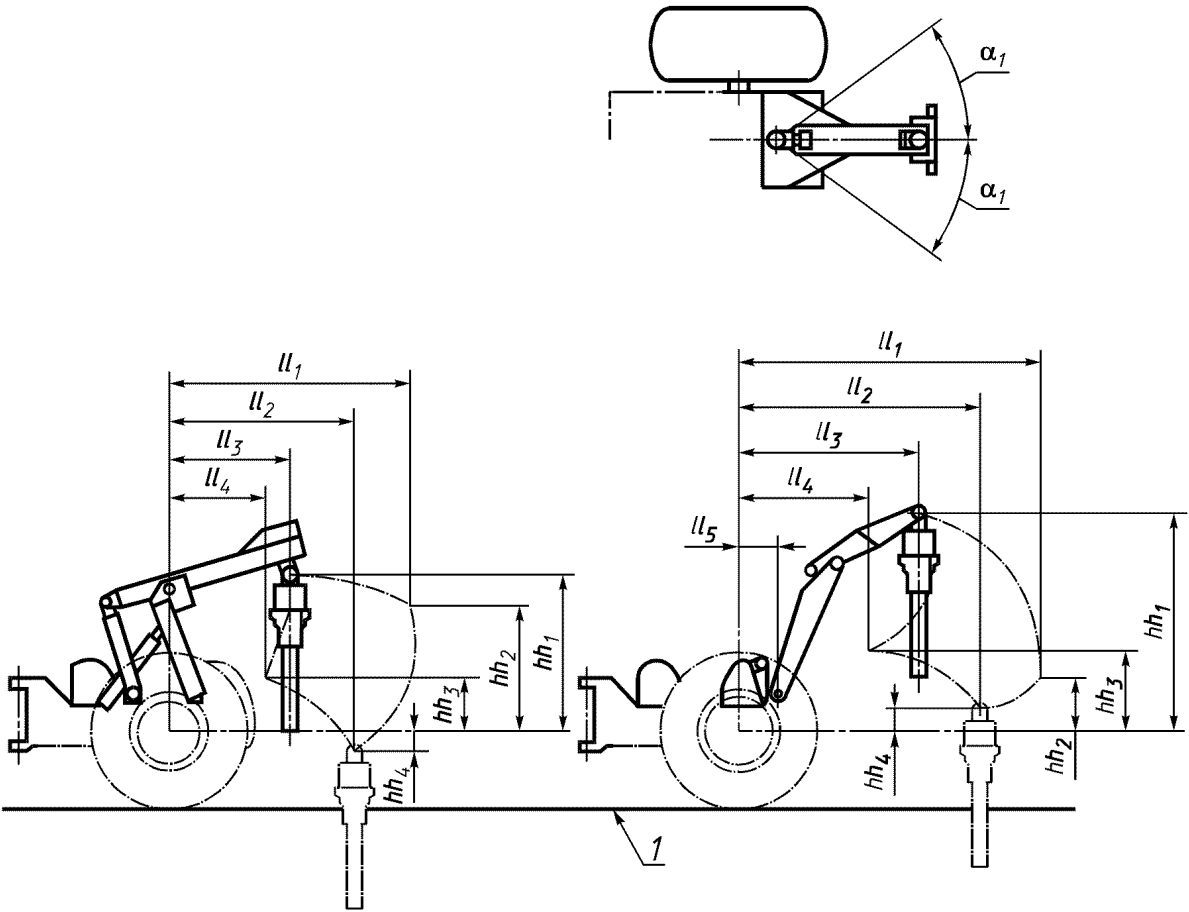
Рисунок 4 — Стрела с захватом
