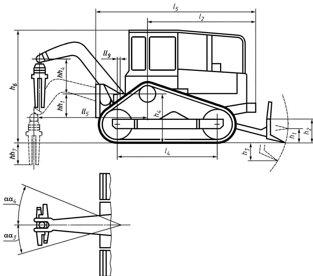
Рисунок 6 — Трелевочная машина с пачковым захватом на базе промышленного шасси. Основные размеры в продольной вертикальной плоскости
