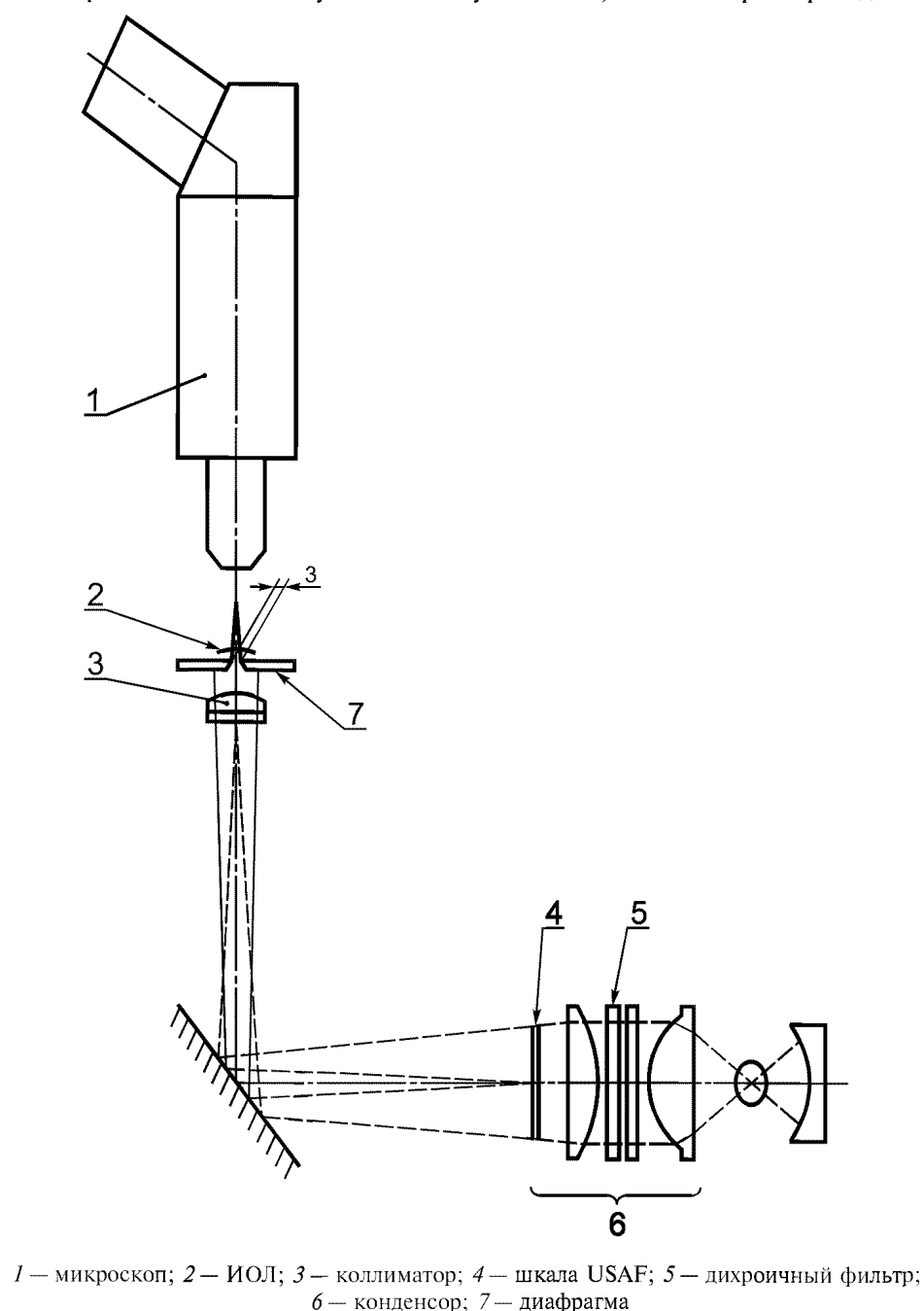
Рисунок А.1 — Оптическая скамья с ИОЛ
