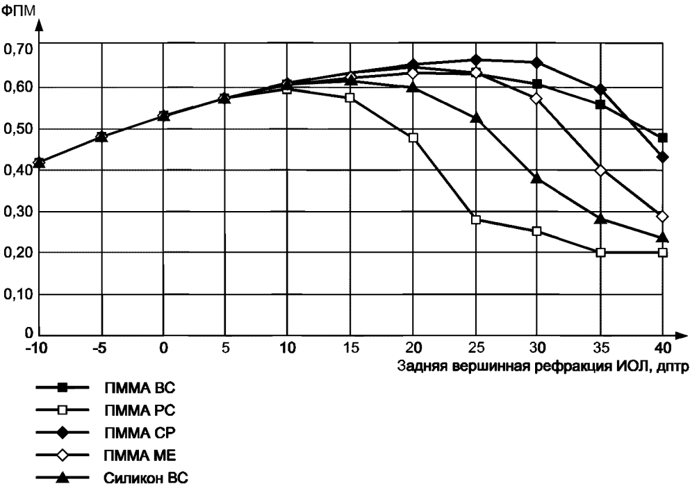
Рисунок В.2 — Рассчитанные значения ФПМ на 100 мм -1 для системы «модель глаза — ИОЛ» различной конструкции
