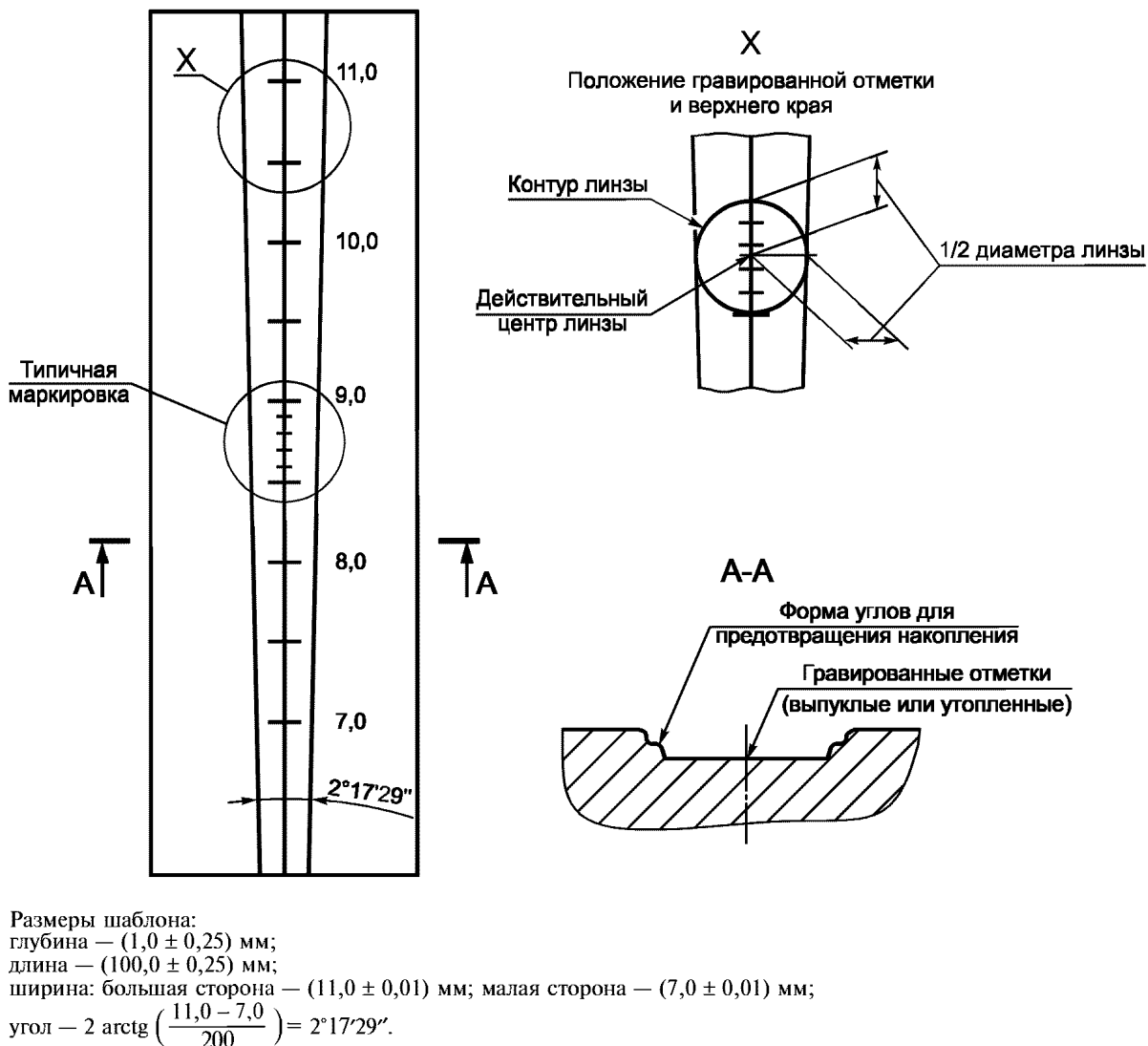
Рисунок Д.1 — V-образный шаблон для измерения диаметра жесткой контактной линзы со шкалой на осевой линии шаблона
