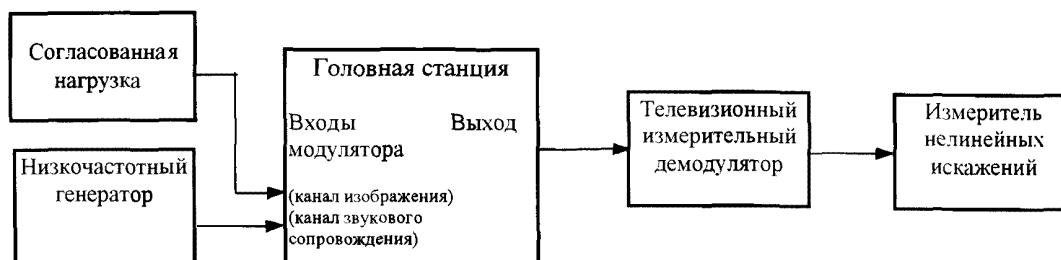
Рисунок 7.26 — Структурная схема для измерения нелинейных искажений сигнала звукового сопровождения
