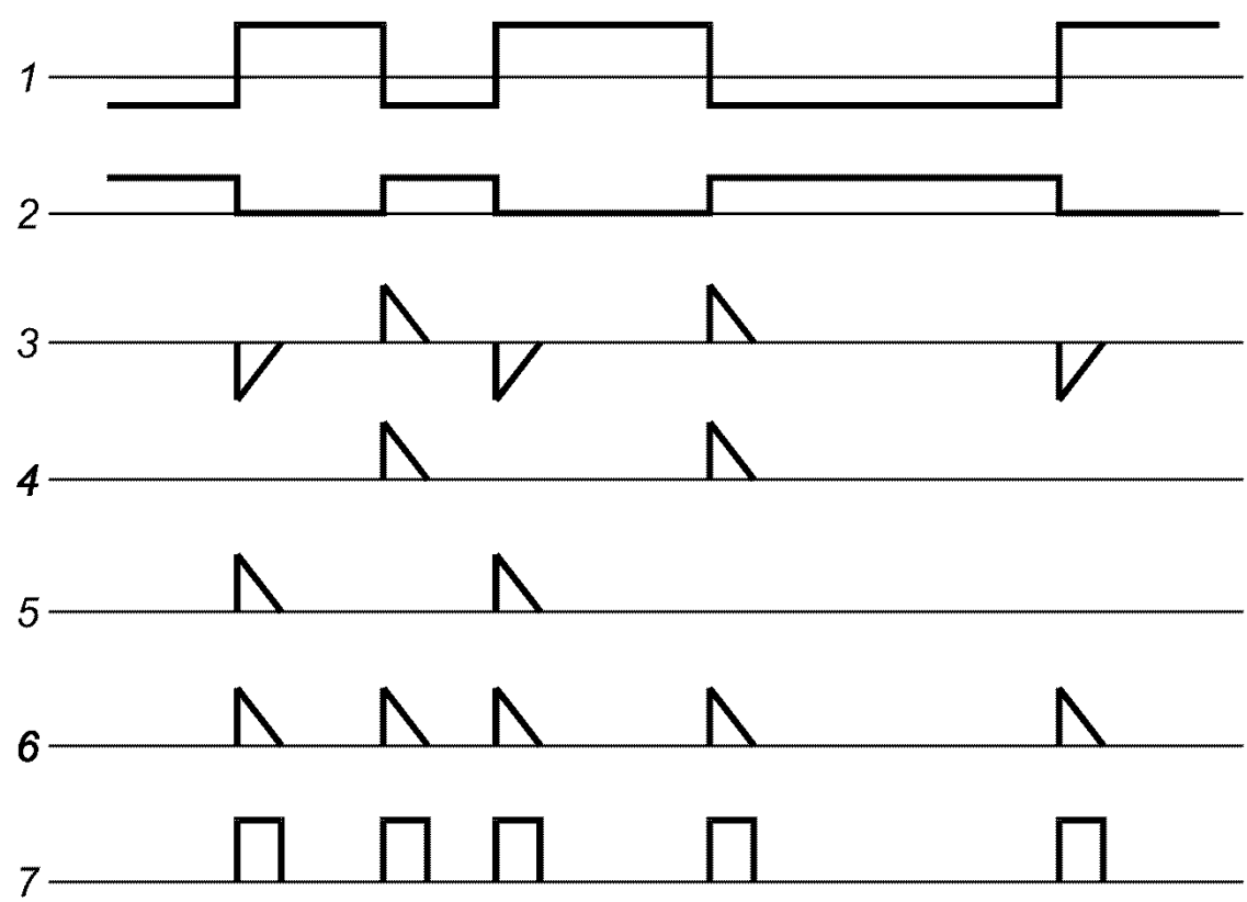
1 — входной сигнал; 2 — сигнал после формирователя однополярного сигнала; 3 — сигнал на выходе дифференцирующей цепи; 4 — неинвертируемые положительные импульсы; 5 — сигнал на выходе инвертора; 6 — сигнал на входе мультивибратора; 7 — выходные импульсы
