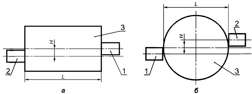
а — Изделия с плоскопараллельными поверхностями б — Изделия с круглыми поверхностями
