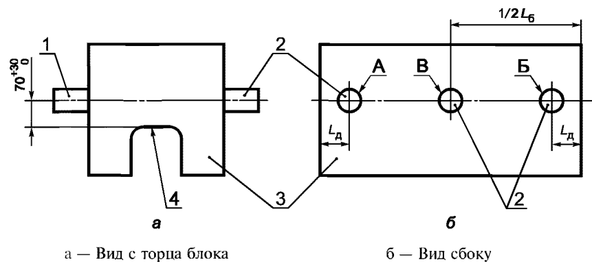
а — Вид с торца блока б — Вид сбоку 1, 2 — электроакустические преобразователи; 3 — блок; 4 — дно паза; L б — длина блока; A, Б, Б* — места контроля; L д — допускаемое расстояние до торца блока
