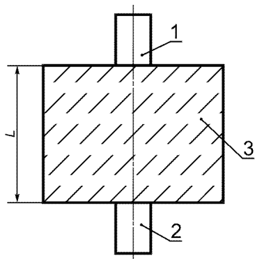
1, 2 — электроакустические преобразователи; 3 — углеродное изделие; L — база прозвучивания
