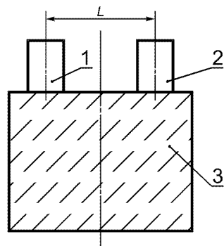
1, 2 — электроакустические преобразователи; 3 — углеродное изделие; L — база прозвучивания
