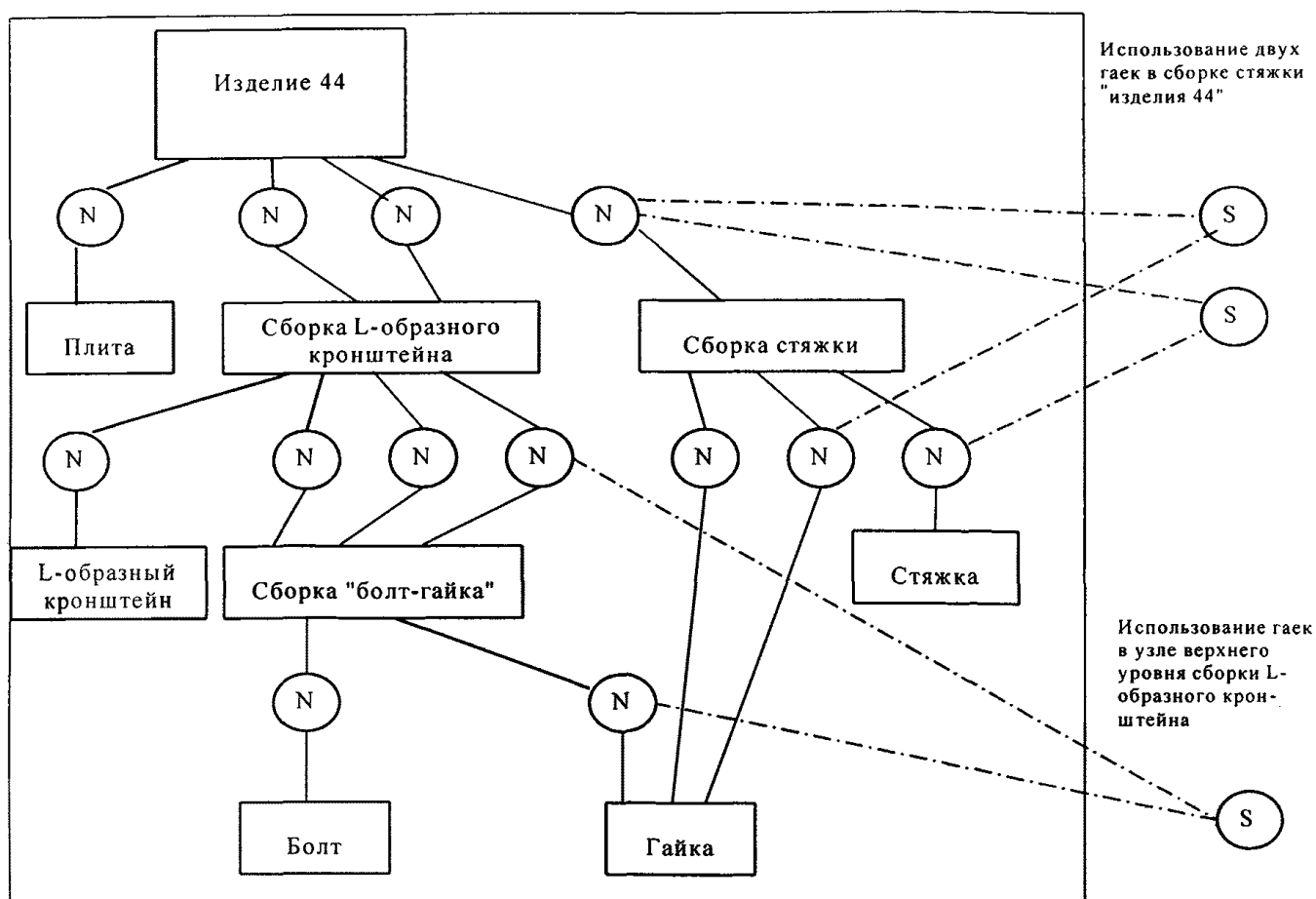
Рисунок Е.9 — Конкретное применение в сборке верхнего уровня
