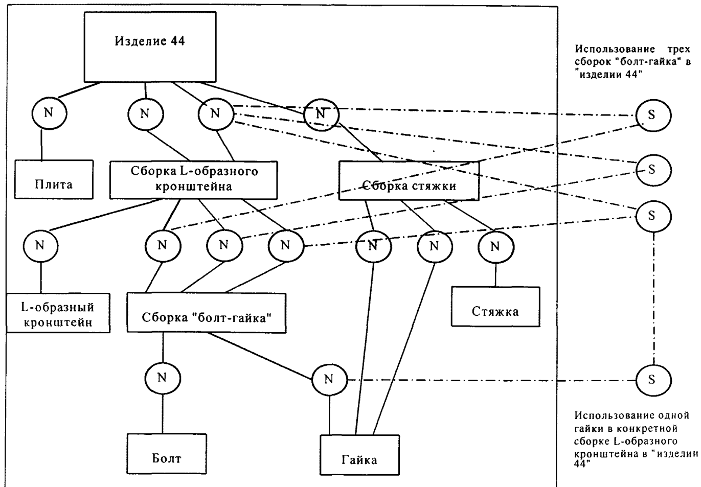
Рисунок Е.10 — Полное применение в сборке верхнего уровня
