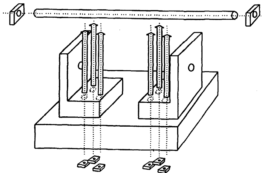
Рисунок Е.1 — Изделие 44
