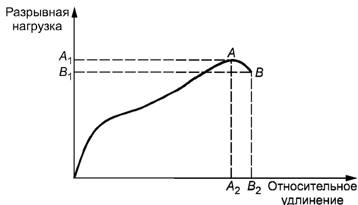
Рисунок 1 — Типичная кривая разрывная нагрузка — относительное удлинение
