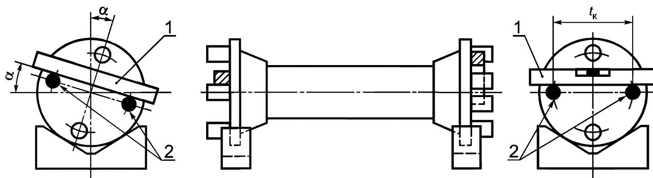
1 — пузырьковый уровень; 2 — центровочные штыри
