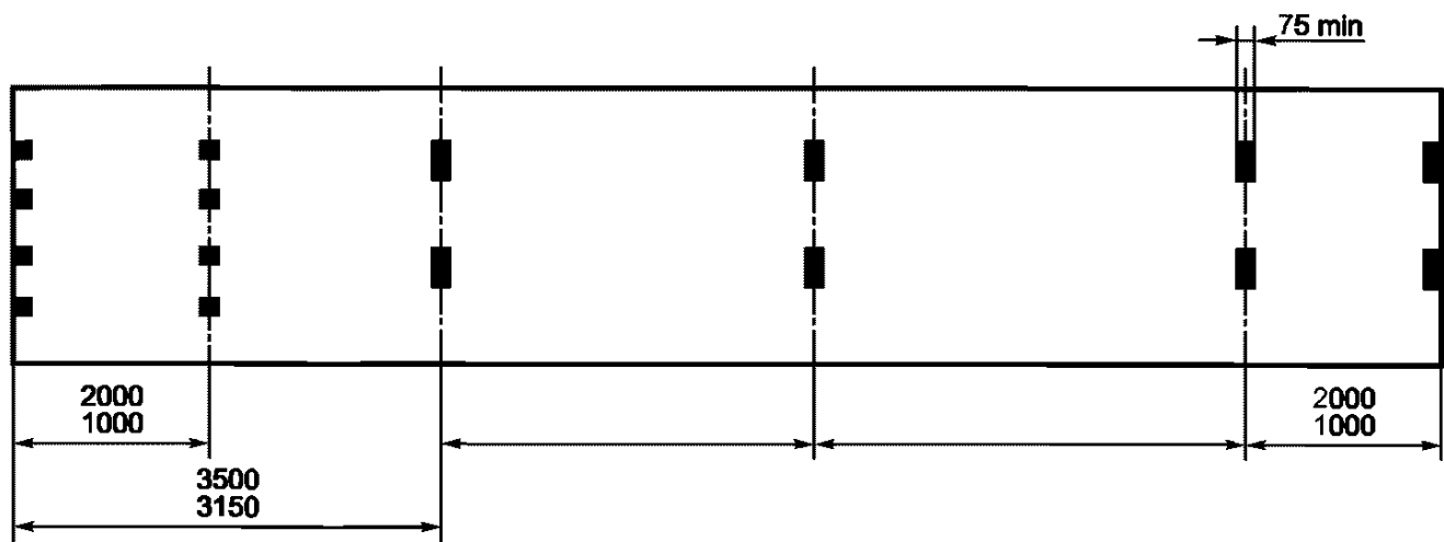
Рисунок Б.4 — Минимальное количество пар опорных (контактных) площадок контейнеров типов 1AAA, 1AA, 1A и 1AX с туннелем для захвата типа «шея гуся»
