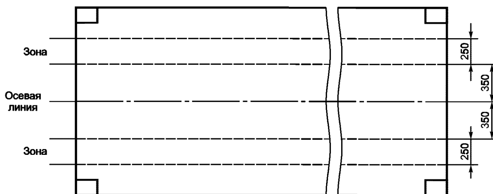
Рисунок Б.1 — Размеры зон в продольном направлении
