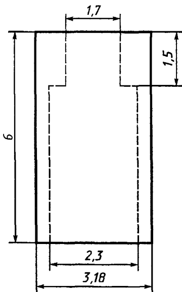
Рисунок R.1 — Кожух датчика
