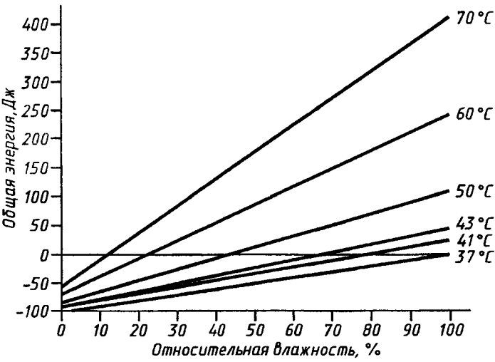
Рисунок S.1 — Передача тепла, поглощенного газом при 37 °С
