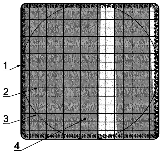
1 — граничный контур (рекомендуемый); 2 — квадратная сетка (обязательная); 3 — вписанная окружность (рекомендуемая); 4 — 50 % среднего уровня изображения (фон)
