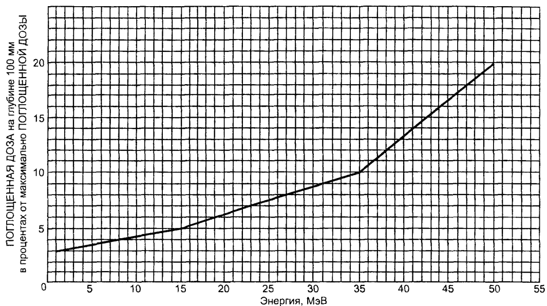
Рисунок 101 — Пределы НЕИСПОЛЪЗУЕМОГО ТОРМОЗНОГО ИЗЛУЧЕНИЯ во время ЭЛЕКТРОННОГО ОБЛУЧЕНИЯ (29.2.1)
