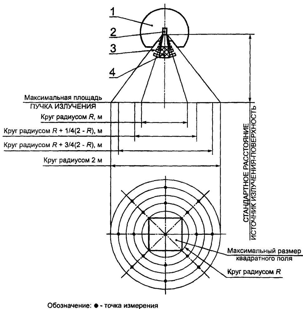
1 — РАДИАЦИОННАЯ ГОЛОВКА; 2 — ИСТОЧНИК ИЗЛУЧЕНИЯ; 3 — УСТРОЙСТВО ФОРМИРОВАНИЯ ПУЧКА; 4 — ЗАЩИТНАЯ ЗАГЛУШКА
