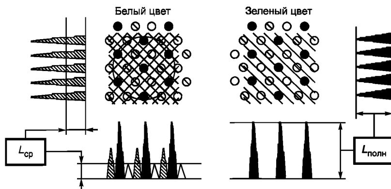
Рисунок Г.2 — Контрольный квадрат для коррекции яркости основного цвета
