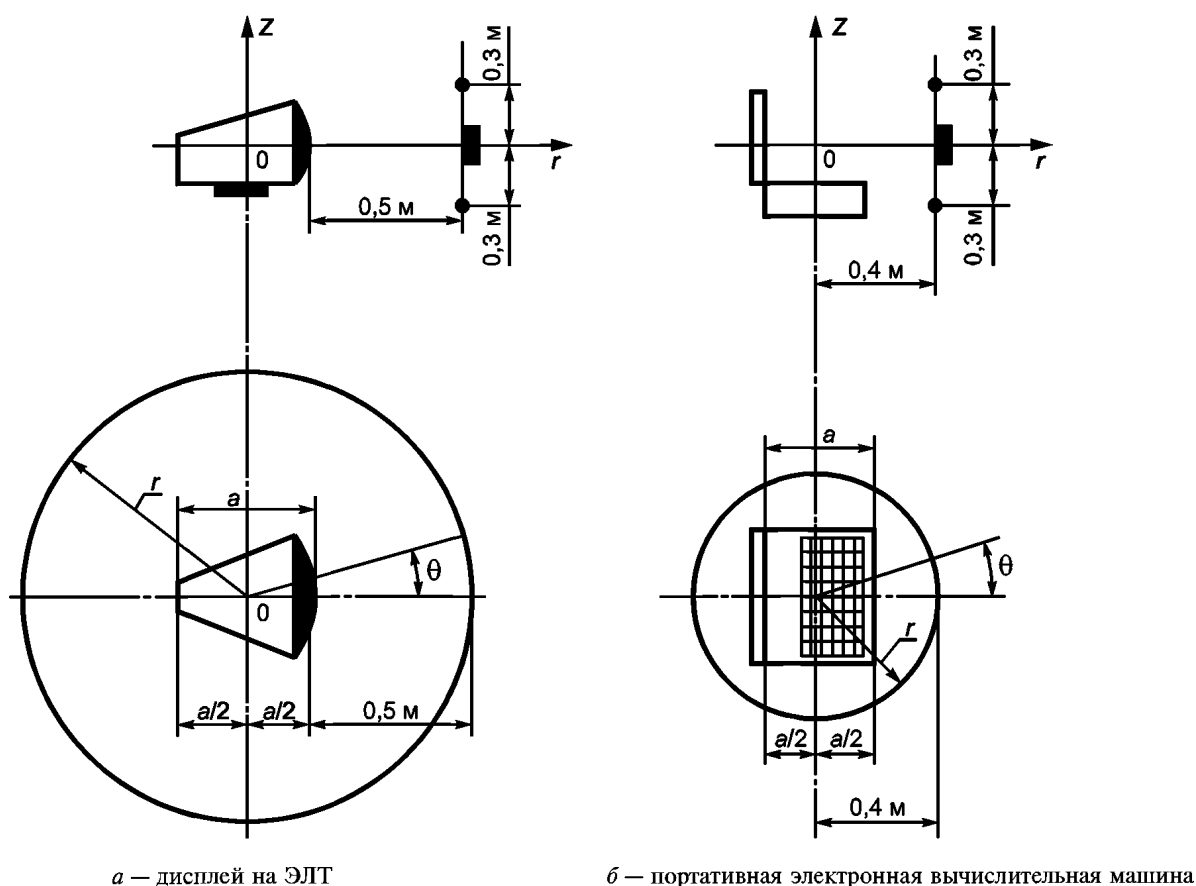
Рисунок 8 — Схема расположения дисплеев в цилиндрической системе координат
