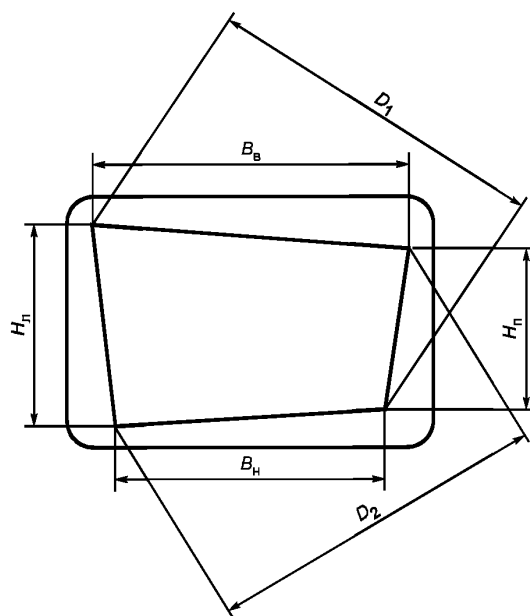
Рисунок 6 — Определение отклонения рабочего поля от прямоугольной формы
