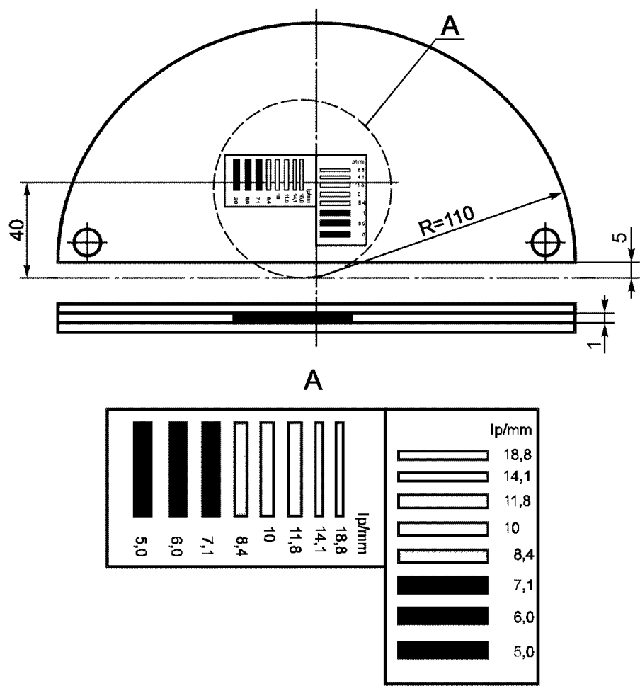
Рисунок 2 — Высококонтрастный ТЕСТ-ОБЪЕКТ (1-й вариант)
