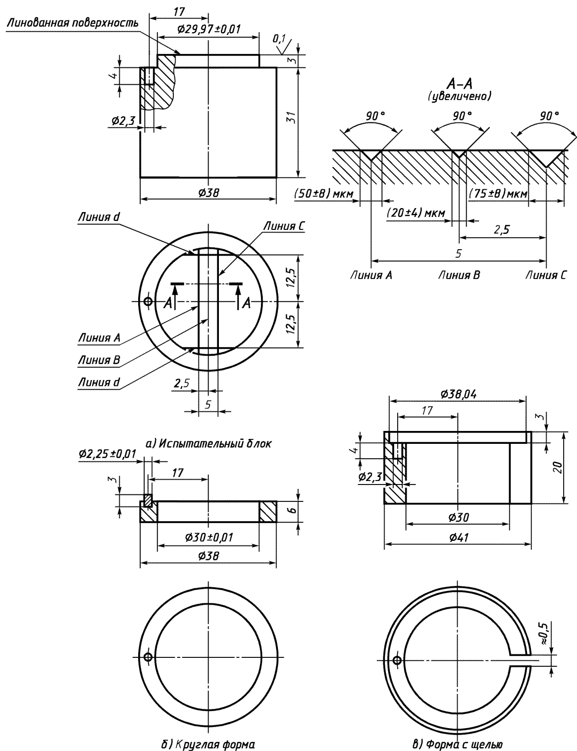
Рисунок 1 — Схема прибора для воспроизведения деталей
