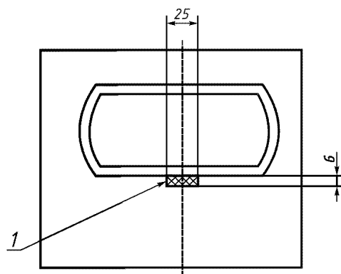
1 — площадка, воспринимающая нагрузку при неправильной установке контейнера
